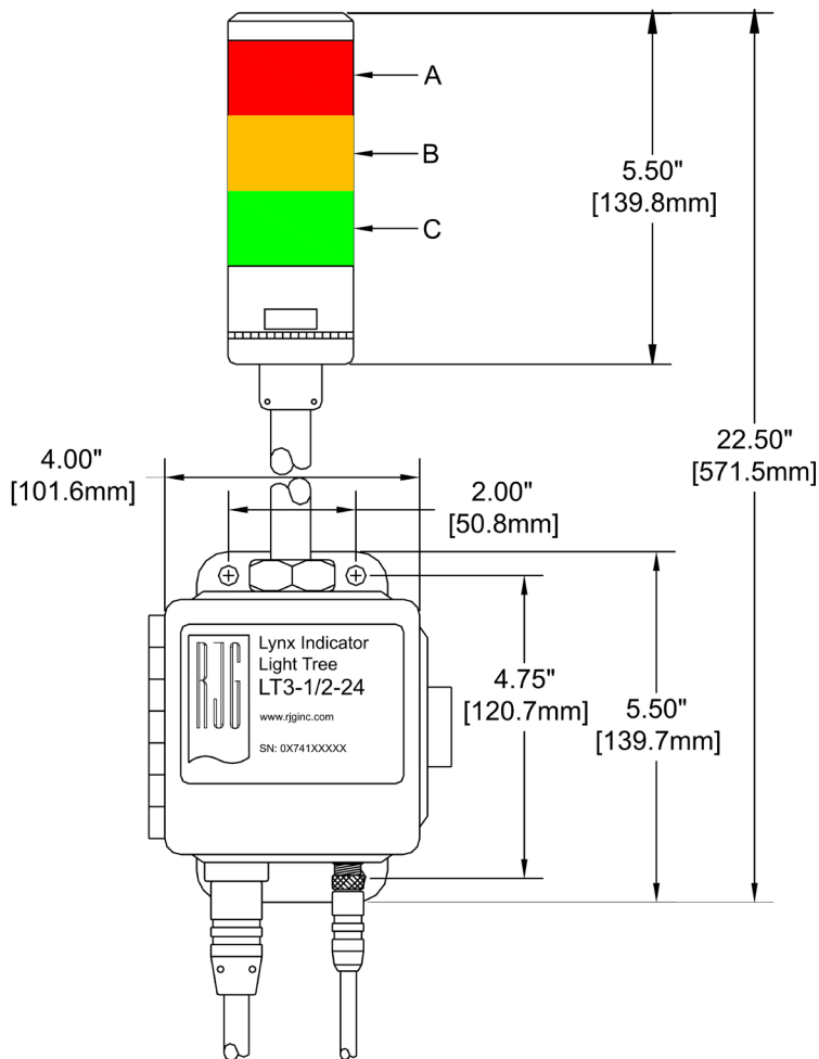
图14: Lynx™ 指示光树 (24 伏直流)
